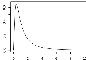
LogNormal(0,1)
