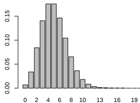
Poisson(5)
